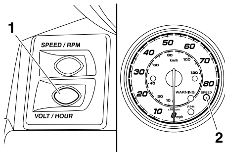
1 "VOLT/HOUR"-Knopf
