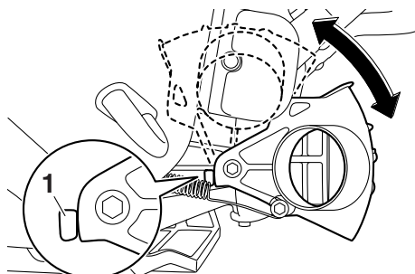
1 Anschlag
