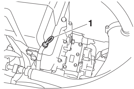
1 Messstab
