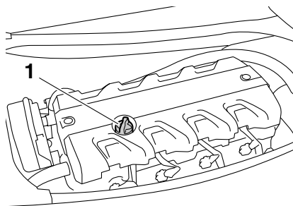
1 Motoröl-Einfüllverschluss
