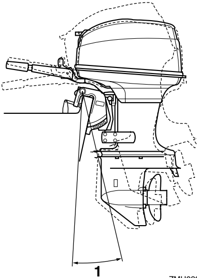
1. Trimbedieningshoek
