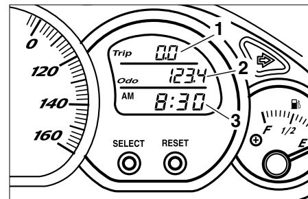
1. Ritteller 2. Kilometer teller, brandstofreserve ritteller 3. Klok, buitentemperatuur display en voltagedisplay
