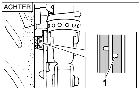
1. Slijtage-indicatiegroef
