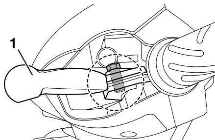
1. Achterremhendel
