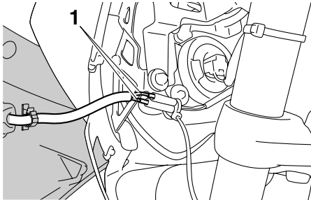
1. Kabelstekker richtingaanwijzer
