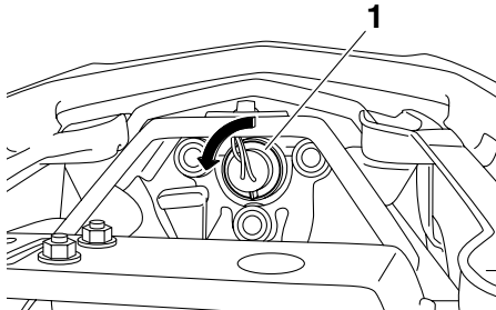
1. Gloeilampfitting remlicht/achterlicht
