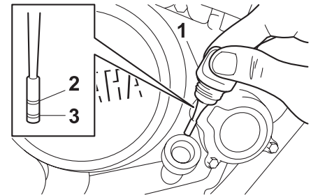
1. Motoröl-Einfüllschraubverschluss
