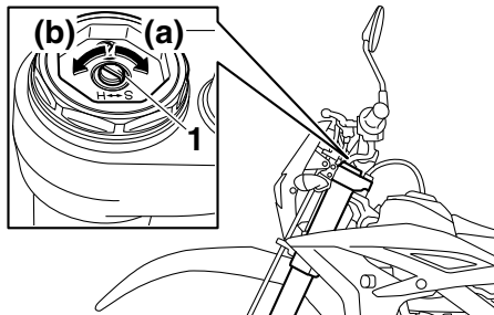
1. Druckstufendämpfungs-Einstellschraube
