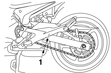
1. Spanning aandrijfketting
