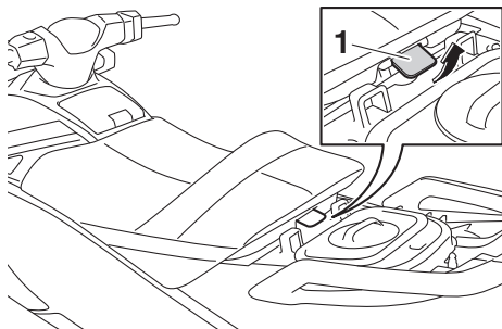
1 Sitzbank-Entriegelungshebel
