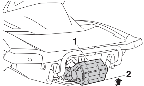
1 Umkehrklappe 2 Neutralstellung
