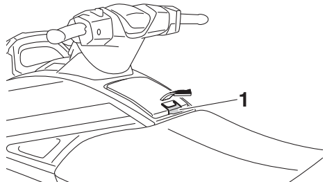
1 Handschuhfach-Entriegelungshebel
