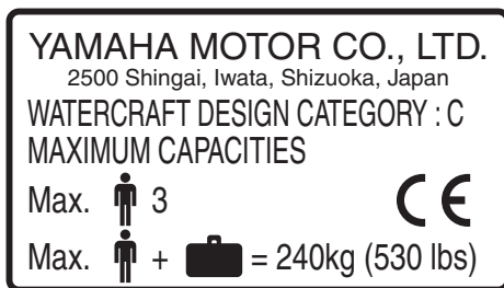
1 Θέση για το πινακίδάκι κατασκευαστή
