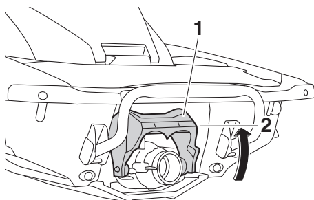
1 Compuerta de inversión 2 Posición de marcha avante
