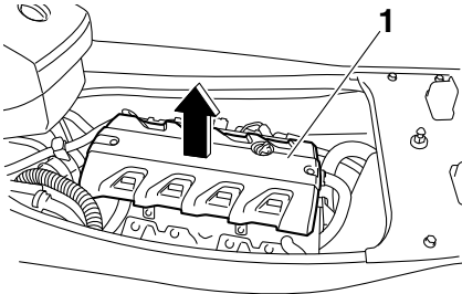
1 Καπάκι κινητήρα
