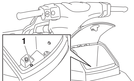
1 Ablassschraube
