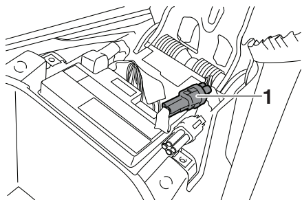
1. Diagnosestekker brandstofinspuiting
