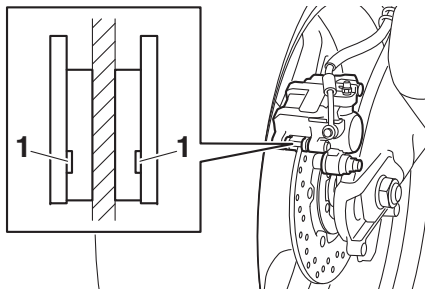
1. Slijtage-indicatorgroef remblok
