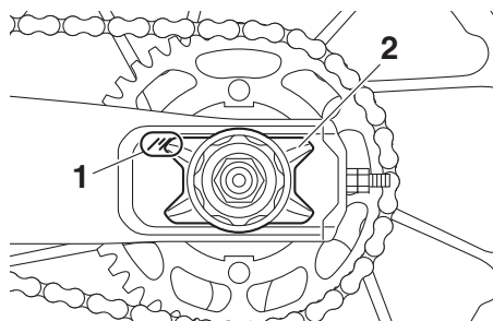
1. Uitlijnermerktekens
