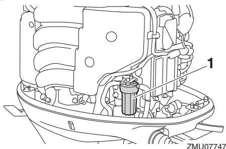
1. Brandstoffilter
