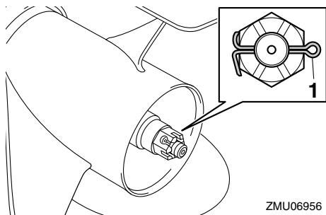
1. Splitpen
