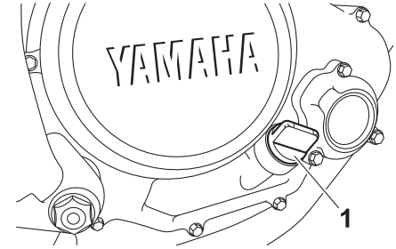
1. Olievuldop
