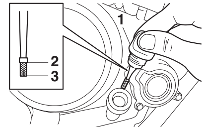
1. Olievuldop
