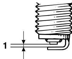
1. Zündkerzen-Elektrodenabstand
