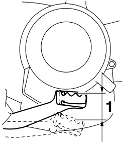
1. Fußbremshebel-Spiel
