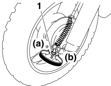
1. Einstellmutter für das Spiel des Handbremshebels
