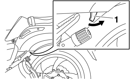
1. Palanca de liberación del respaldo del asiento del conductor
