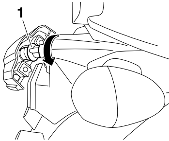
1. Gloeilampfitting kentekenverlichting
