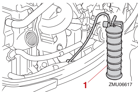
1. Olieverser
