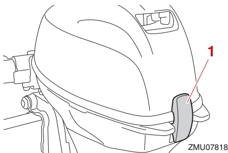
1. Motorkapvergendelhendel
