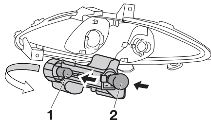
1. Gloeilamp richtingaanwijzer 2. Gloeilamp remlicht/achterlicht
