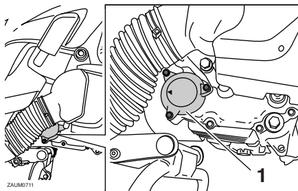
1. Oliefilterdeksel
