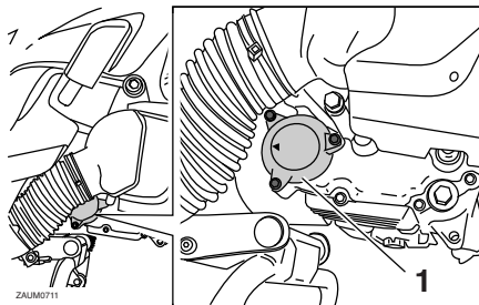
1. Oliefilterdeksel
