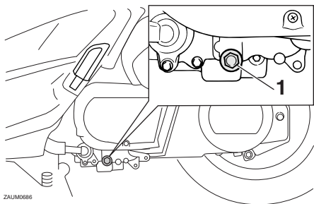
1. Olieaftapplug
